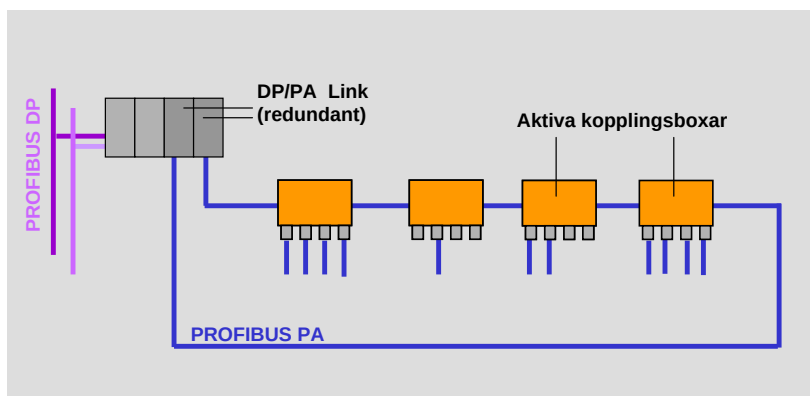
Bild 6: PA ringredundans
