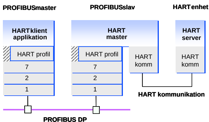
Bild 12: HART-enheter som kommunicerar över PROFIBUS
